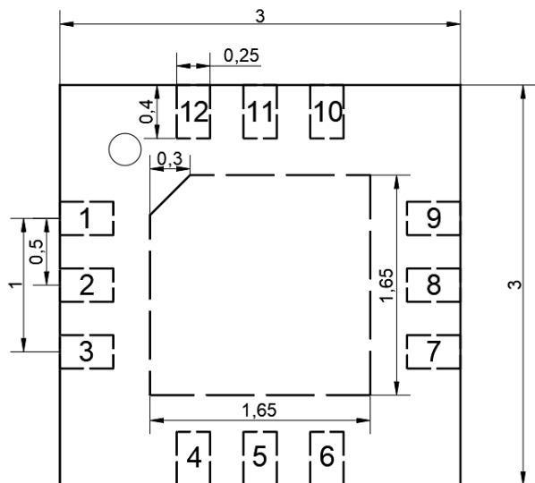
俯视透视图
